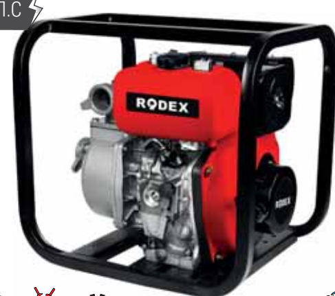
Ручной/Электрический Стартер 4-тактный двигатель Датчик масла 100 мм (4") Диаметр Дизельный Двигатель
